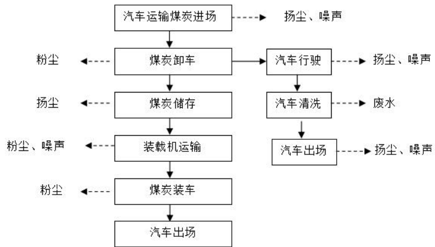
图 2-4 储煤工艺流程图
