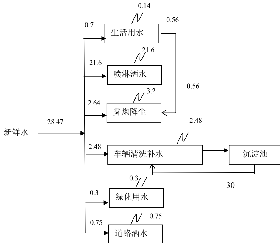
图 2-1 非采暖期水平衡图 (m 3 /d)
