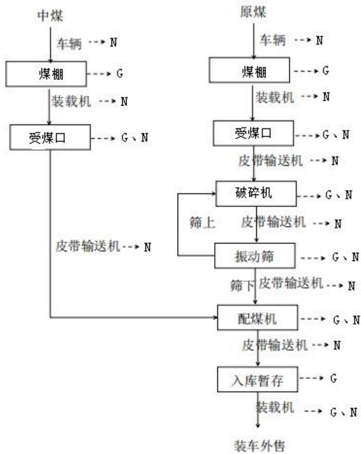
图 2-5 配煤工艺流程图
