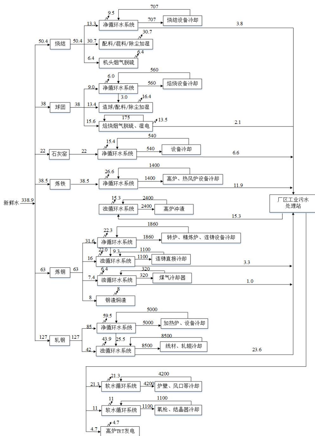
图 3.2.1-4 本项目建成后全厂水平衡图（单位：m³/h）
