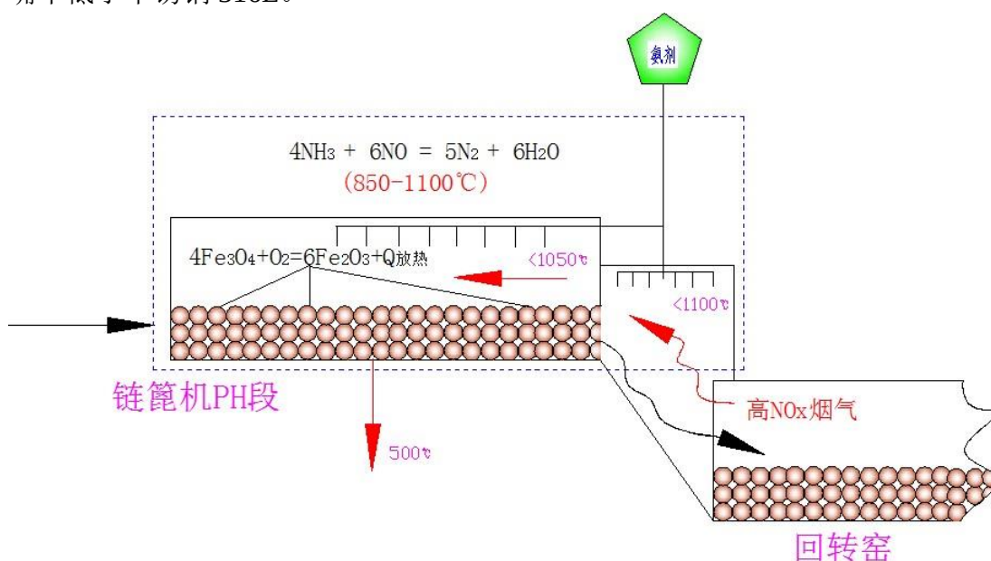
图 6.2.1-3 SNCR 喷射系统布设位置
