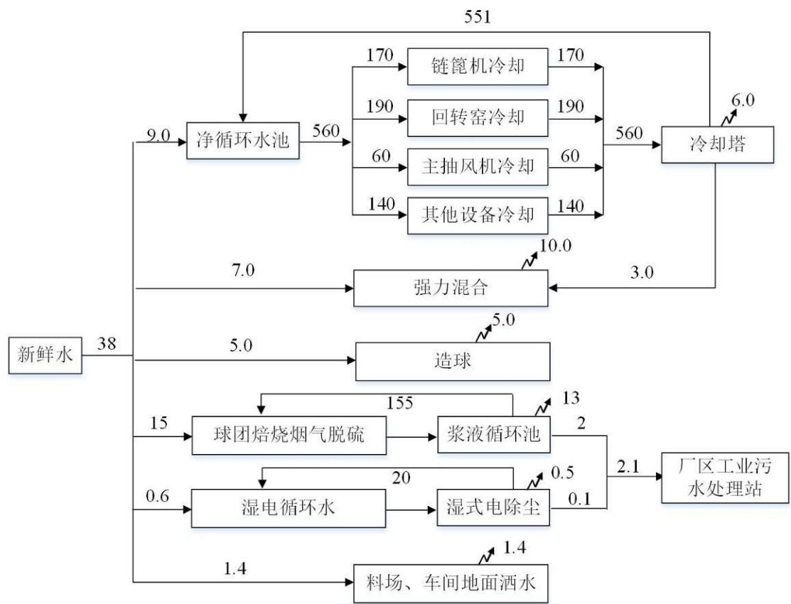
图 3.2.1-3 本项目水平衡图 (单位: m 3 /h)
