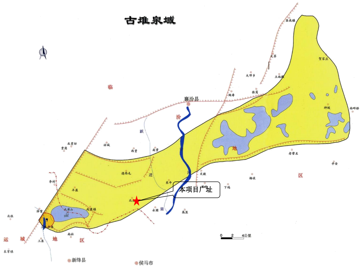
图 4.2.2-1 本项目与古堆泉域位置关系图
