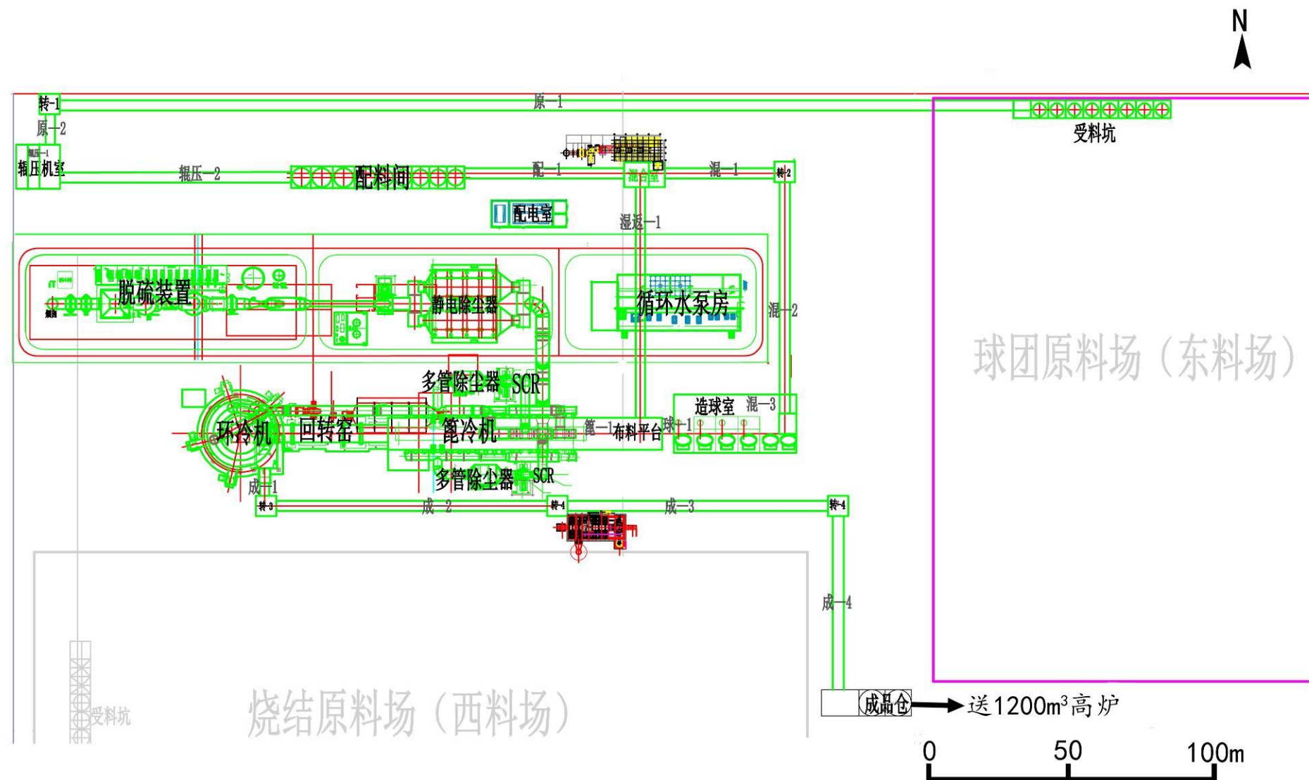
图 3.2.1-1 本项目平面布置图
