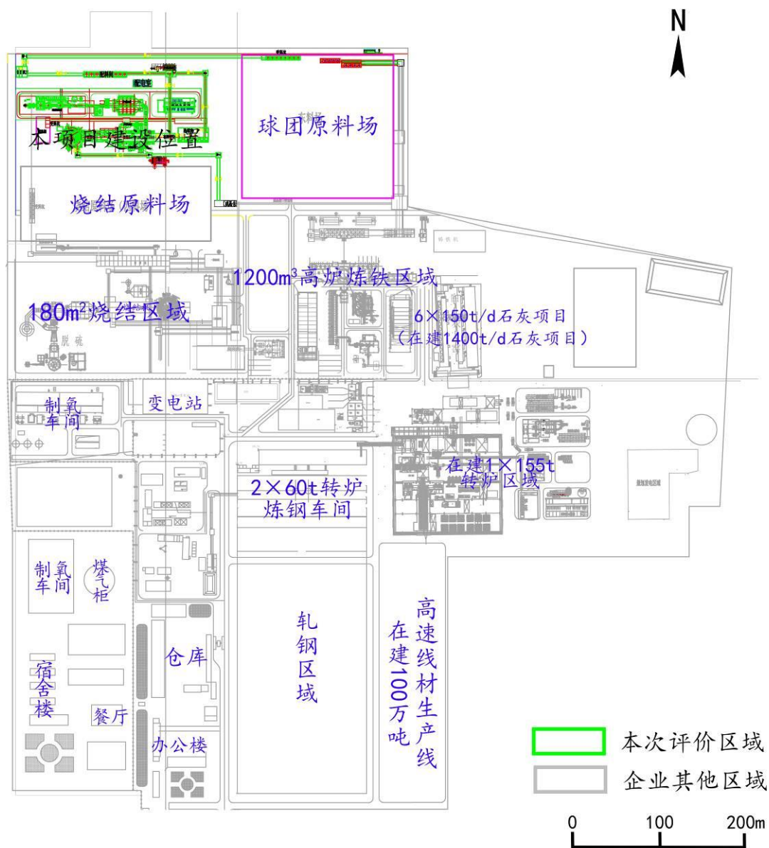
图 3.2.1-2 本项目建成后全厂平面布置图
